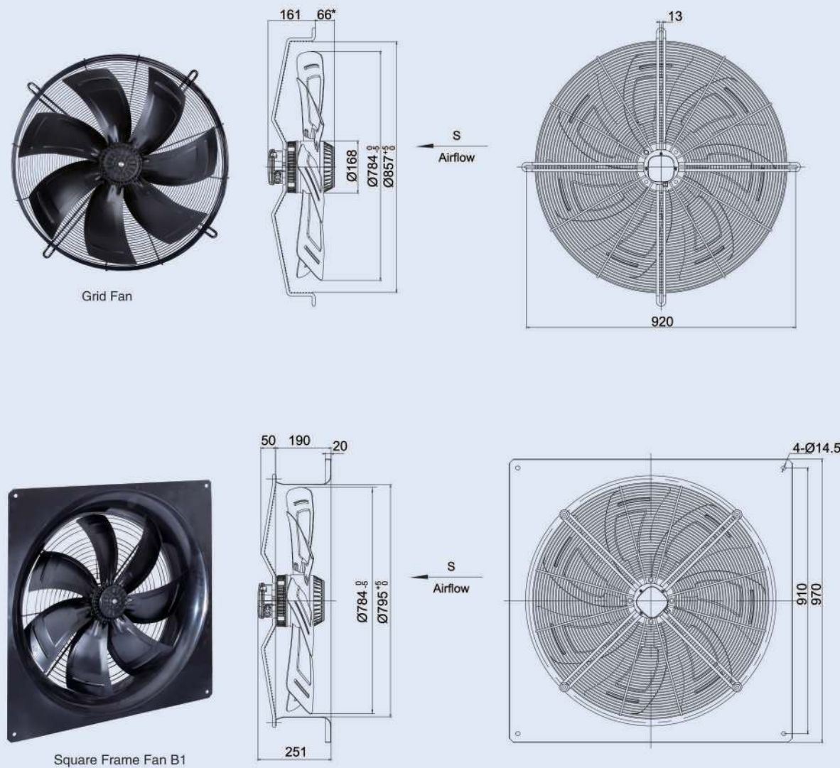
Square Frame Fan B1
